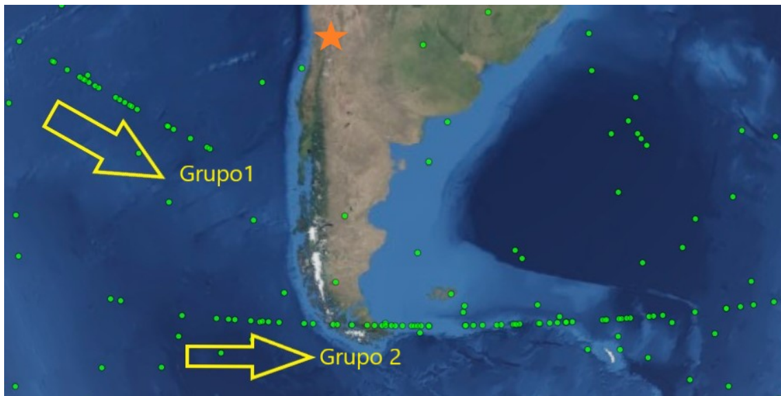
Figura 3. Tránsitos aeroespaciales de las 18:56 del 29 de abril de 2021. Una estrella naranja marca la ubicación del usuario. Flechas amarillas muestran la dirección y sentido del desplazamiento de los satélites. Imagen recortada, no se muestra a todo el Grupo 2.
